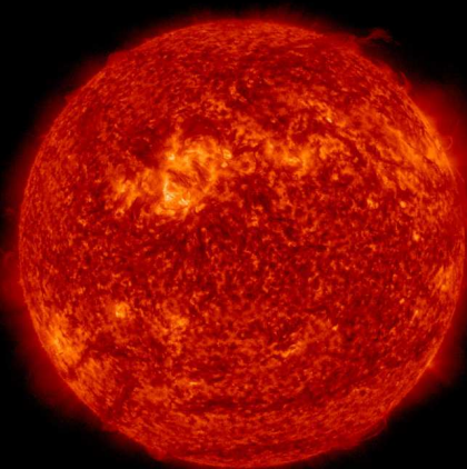
SDO/AIA 304 2022-11-09 16:28:18 UT
