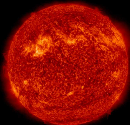
SDO/AIA 304 2022-11-08 18:13:42 UT
