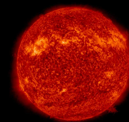
SDO/AIA 304 2022-11-07 18:28:06 UT
